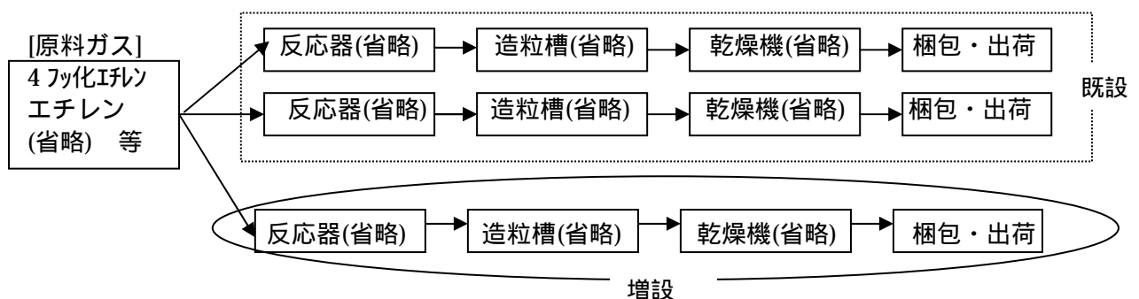
【施設概念図】
