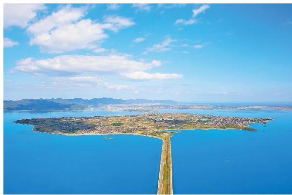
中海に浮かぶ大根島
