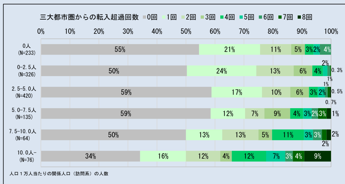
図 17 人口 1 万人当たりの関係人口（訪問系）の人数と三大都市圏からの転入超過回数
