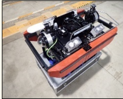
栈橋上部工下面の 点検診断ロボット
