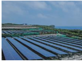
島南部の七又海岸の約10万m 2 の敷地に、総出力4,000kWの太陽光発電設備を設置。年間発電量は一般家庭約1,200世帯分の電気使用量に相当する。
