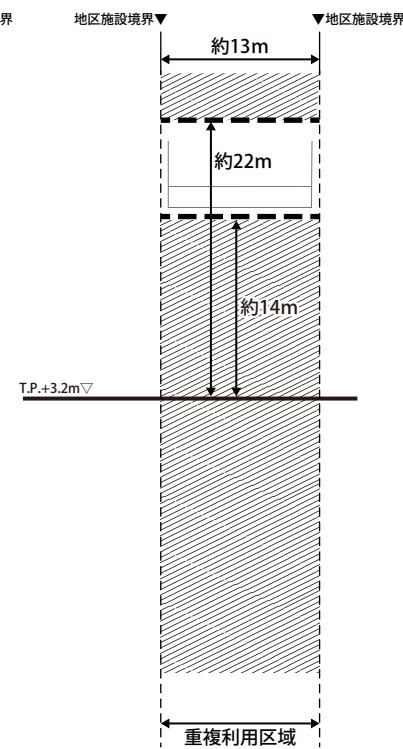
C-C'断面
