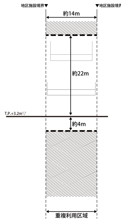
B-B'断面
