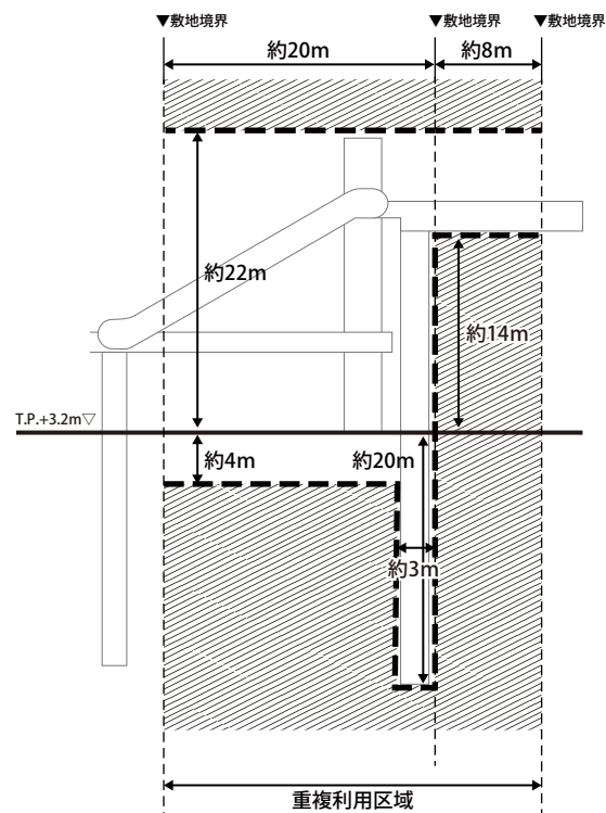
A-A'断面
