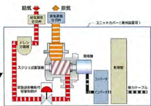
スクルータービン機器構成
