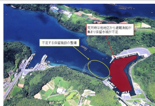
係留施設の整備全体図
