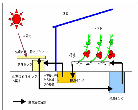
光触媒を使った栽培イメージ図
